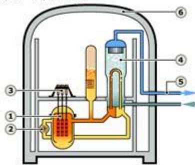
راکتور آب (آب فشرده)
